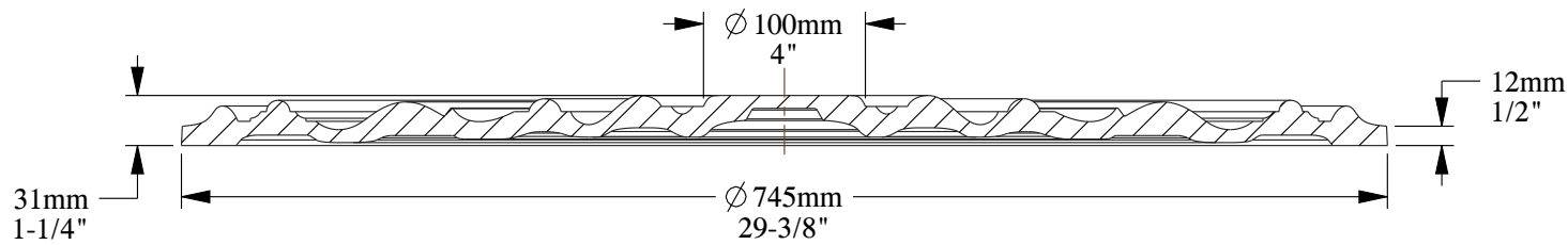
SECTION A-A SCALE 1:5
